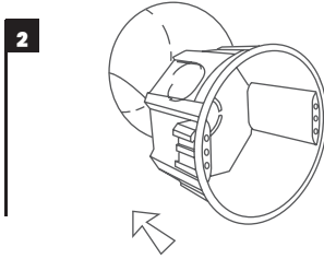
(CZ) Umístěte krabičku (KU-68) do výřezu. (EN) Place the box (KU-68) in the cutout.
