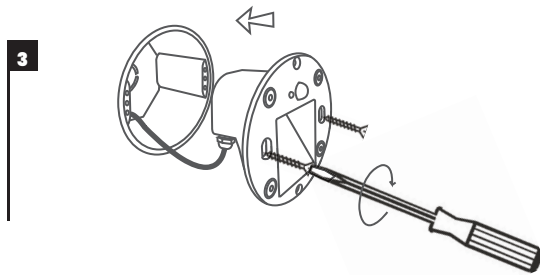
(CZ) Připojte vodič, zatlačte ho do spodní krabice a upevněte jej šrouby. (EN) Connect the wire, push it into the bottom box and fix it with screws.
